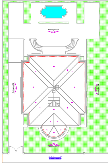
Implantação e Cobertura
