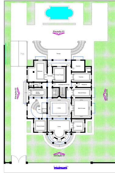
Térreo A = 442,98 m 2
